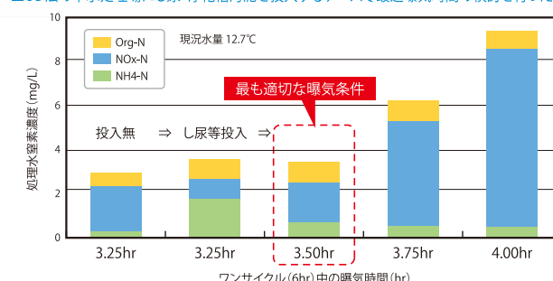
■OD法の下水処理場にし尿・浄化槽汚泥を投入するケースで最適曝気時間の検討を行った事例
