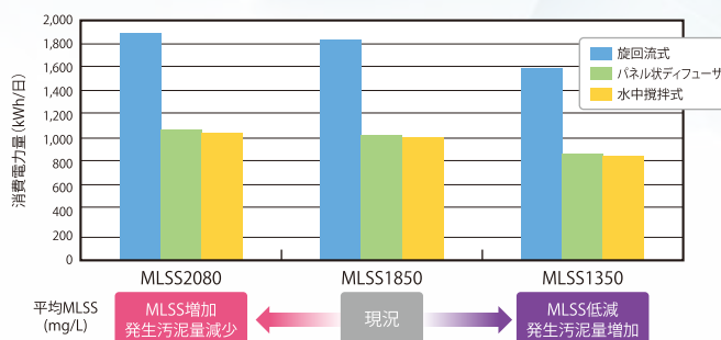
■反応タンクを対象に、各曝気攪拌方式別に、MLSSと消費電力量の検討を行った事例
