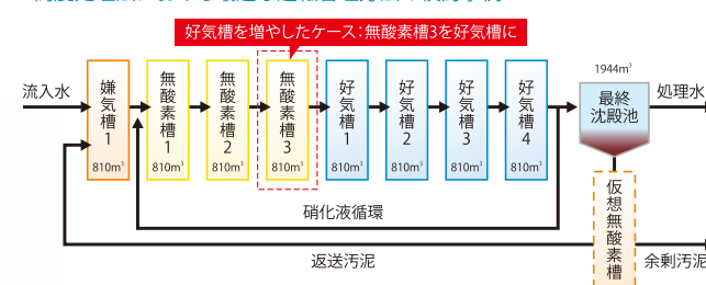
■高度処理法における最適な運転管理方法の検討事例
